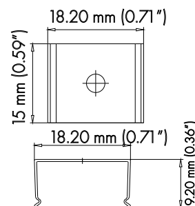
METAL CLIP
